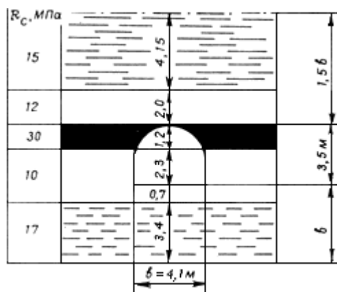
Рис.33. Расчетная схема к примеру 22
