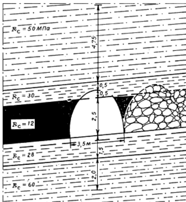
Рис.26. Расчетная схема к примеру 4
