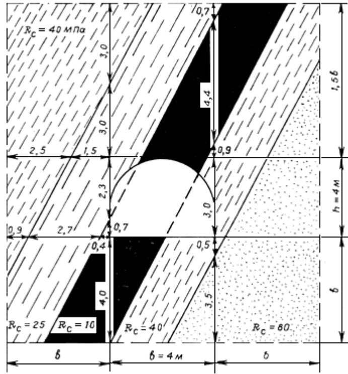
Рис.32. Расчетная схема к примеру 10
