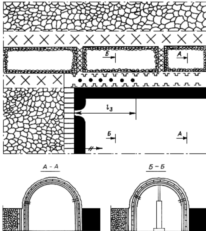
Рис.29. Схема поддержания спаренных выработок, разделенных породной полосой, выкладываемой во время их проходки
