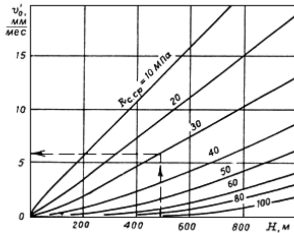
Рис.14. Скорости смещений пород кровли в присечных выработках
