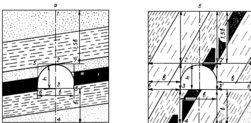
Рис.1. Схемы к определению расчетного сопротивления пород сжатию:
