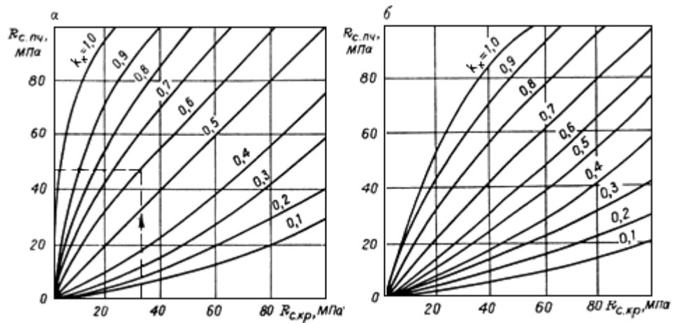
Рис.5. Графики для определения коэффициента k_{к} :
