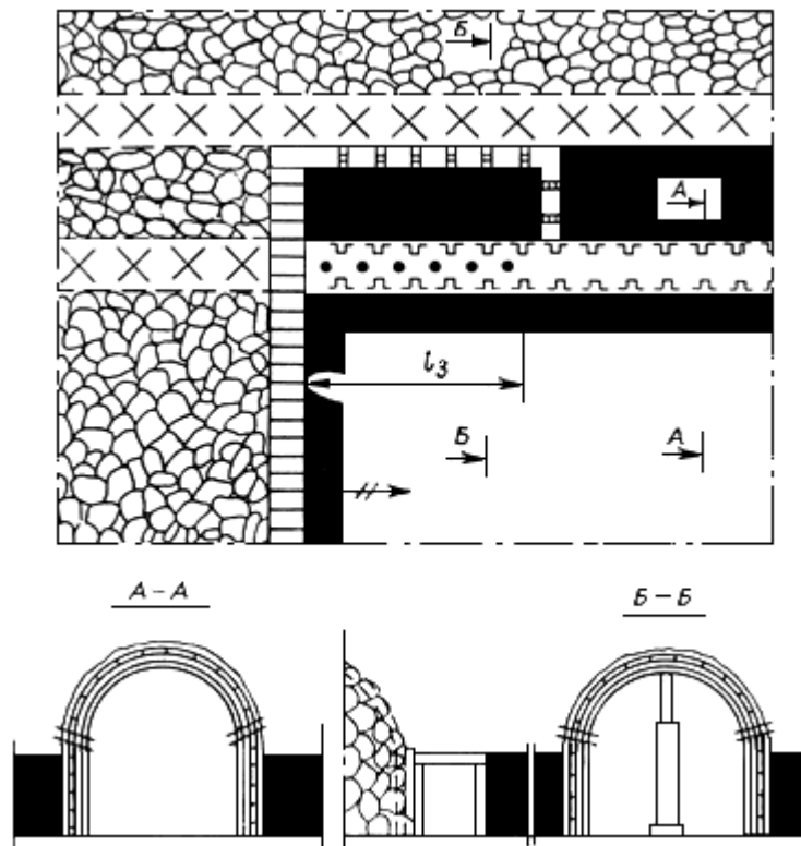
Рис.28. Схема поддержания спаренных выработок, которые разделяет целик угля, извлекаемый одновременно с очистным забоем
