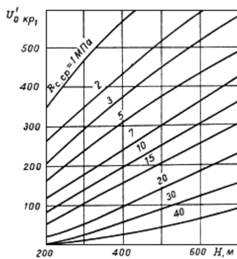
Рис.20. Смещения пород кровли в присечной выработке за первый год ее службы на глубинах:
