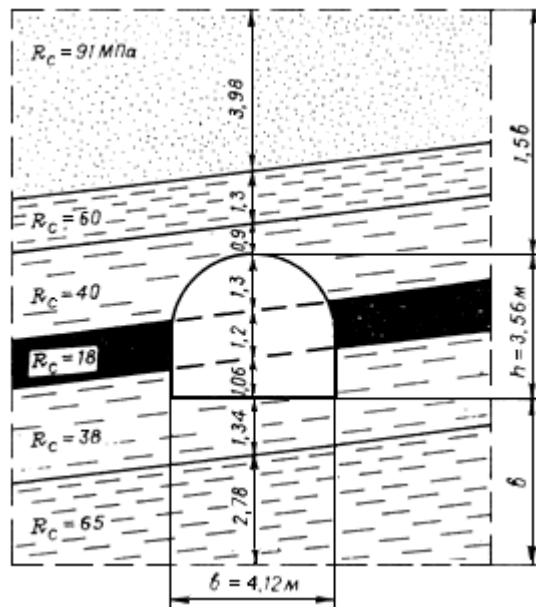
Рис.23. Расчетная схема к примеру 1
