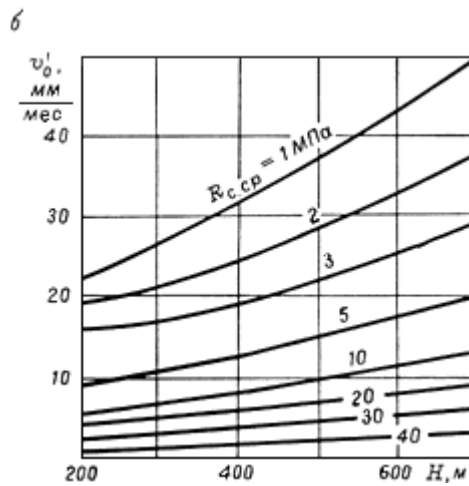
Рис.21. Скорость смещения пород кровли в присечной выработке на глубинах:
