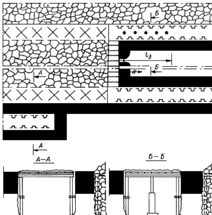
Рис.25. Схема проведения выработок вприсечку к выработанному пространству
