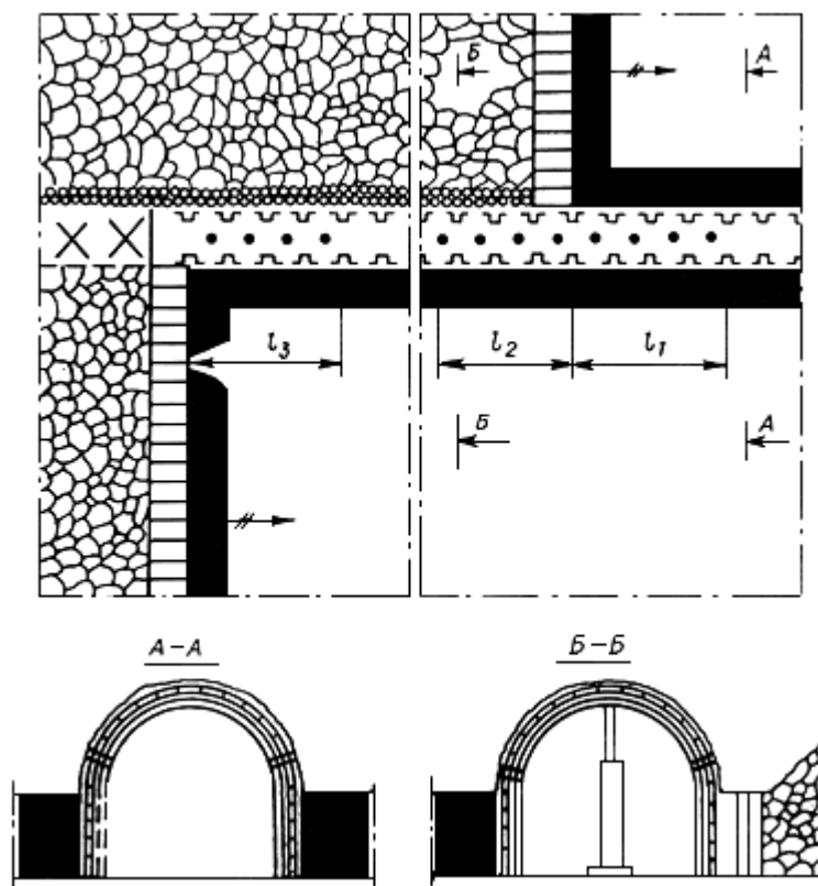
Рис.27. Схема расположения выработок, сохраняемых для повторного использования
