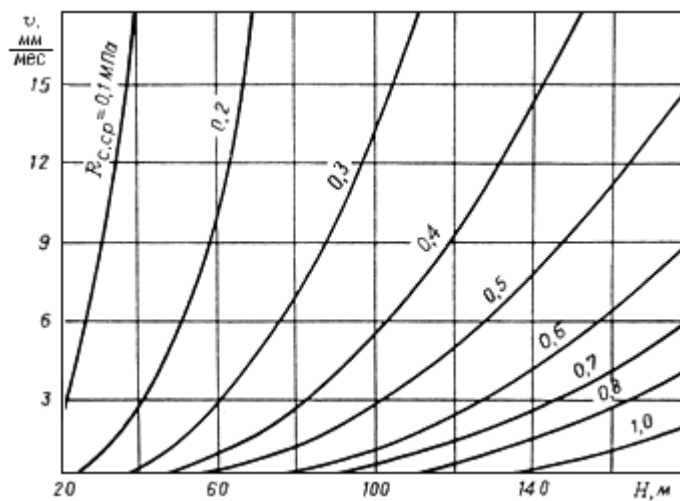
Рис.18. Скорость смещения пород бурого угля месторождений на глубине до 200 м
