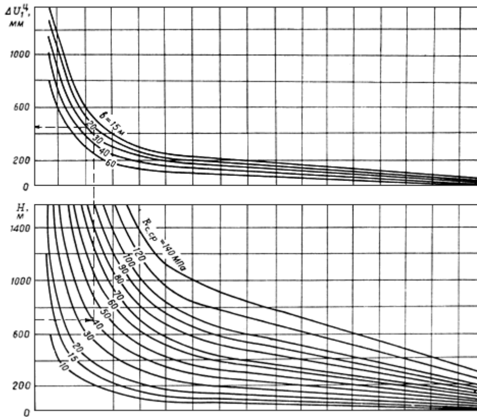
Рис.10. Номограмма для определения \Delta U_1^{II}
