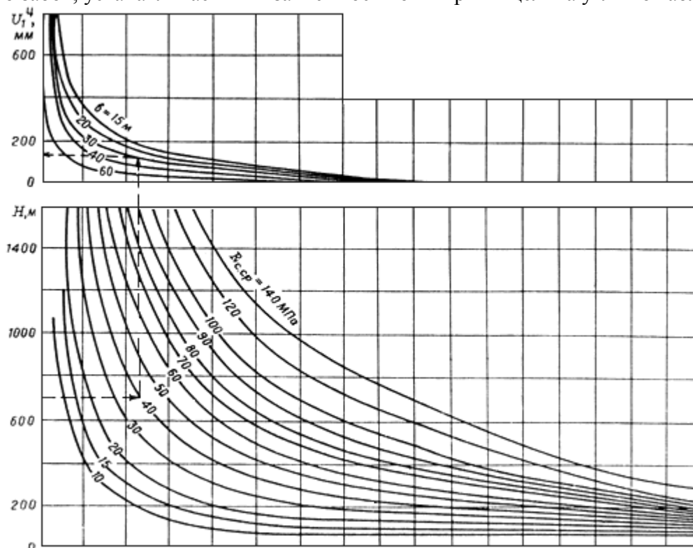
Рис.9. Номограмма для определения U_1^{II}
