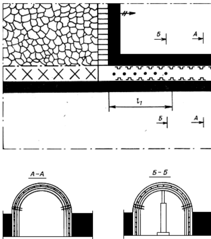
Рис.24. Схема охраны выработок, поддерживаемых в массиве угля в зоне опорного давления очистного забоя
