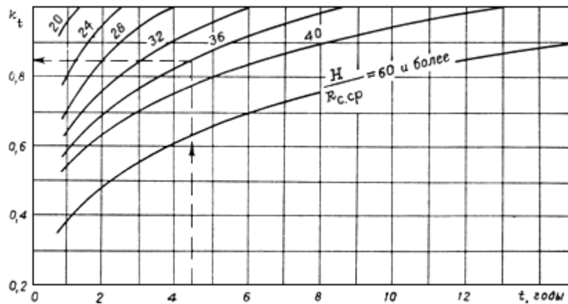
Рис.3. График для определения k_t
