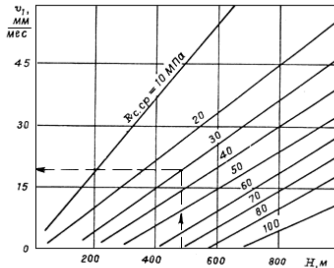
Рис.12. Скорость смещений пород позади очистного забоя
