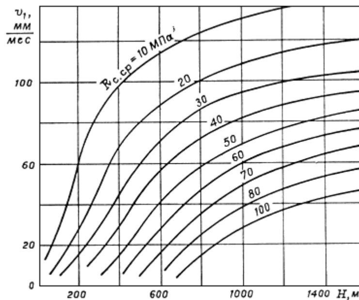
Рис.34. Скорость смещения пород в зоне влияния остаточного опорного давления в выработках, охраняемых искусственными ограждениями
