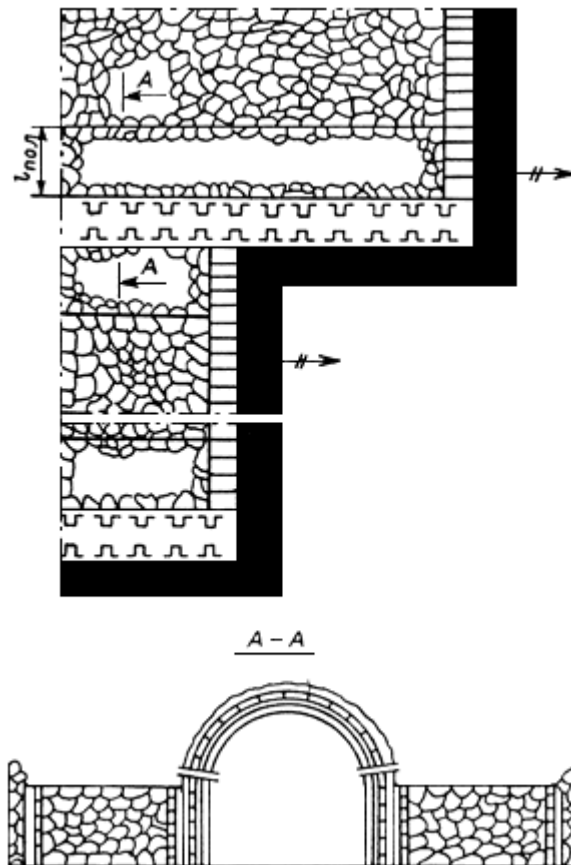
Рис.31. Схема расположения выработок, проводимых (оформляемых) за очистным забоем и сохраняемых для повторного использования
