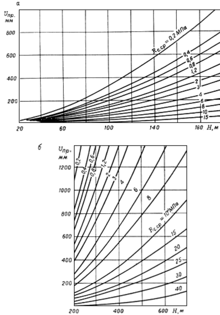
Рис.16. Смещения пород кровли за первый год поддержания выработки на глубинах:
