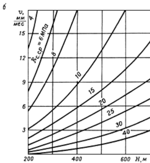
Рис.17. Скорость смещения пород месторождений на глубинах:
