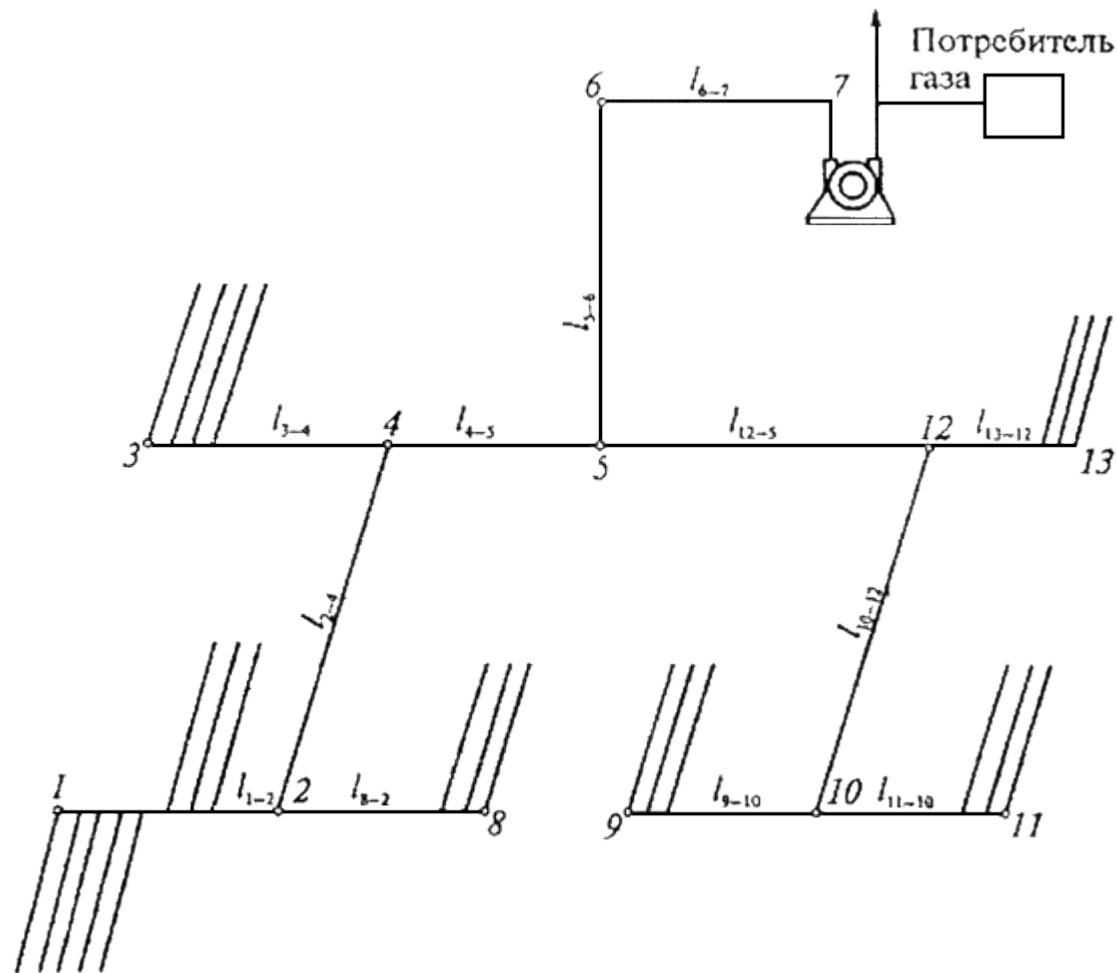
Рис.1. Пример дегазационной сети с древовидной топологией
