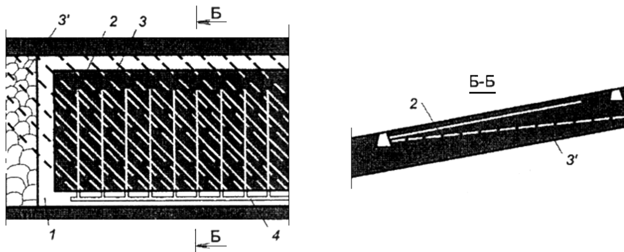
Рис.14. Схема дегазации мощного пласта восстающими скважинами, пробуренными из выработки верхнего слоя:
