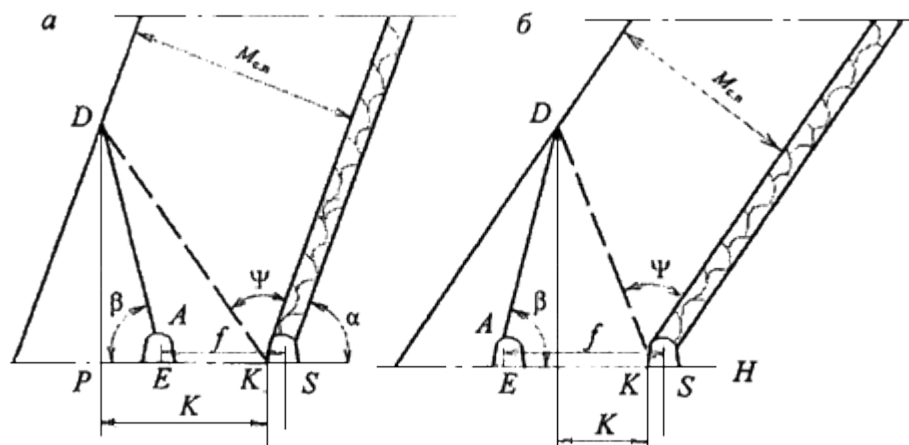
Рис.2. Схема к определению направления скважины, буримой из группового откаточного штрека на вышележащий сближенный пласт, в плоскости, нормальной к простиранию пласта при отсутствии целика угля (бутовой полосы) над штреком:
