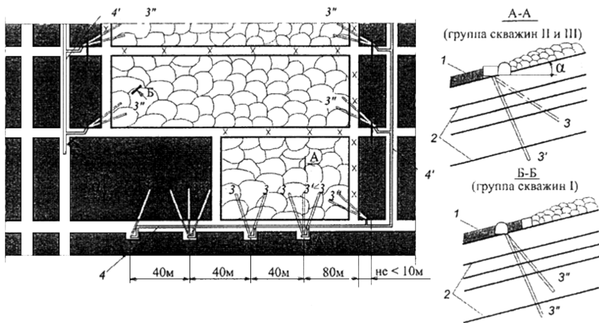
Рис.4. Схема дегазации надрабатываемых пластов скважинами, пробуренными веером из выработок выемочного поля:
