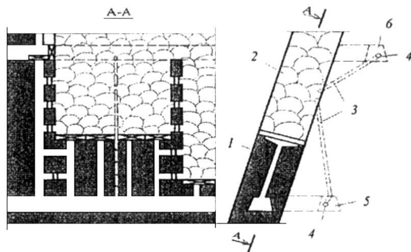
Рис.2. Схема дегазации выработанных пространств мощных крутых пластов скважинами, пробуренными из полевых выработок:
