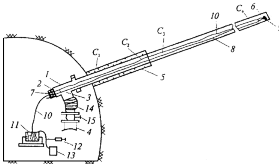
Рис.1. Схема устройства и применения зонда для измерения содержания метана в скважине
