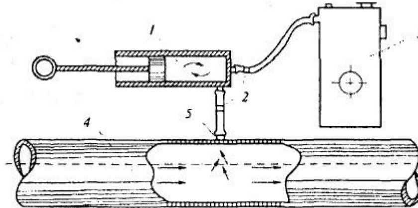
Рис.2. Схема отбора проб газовой смеси:
