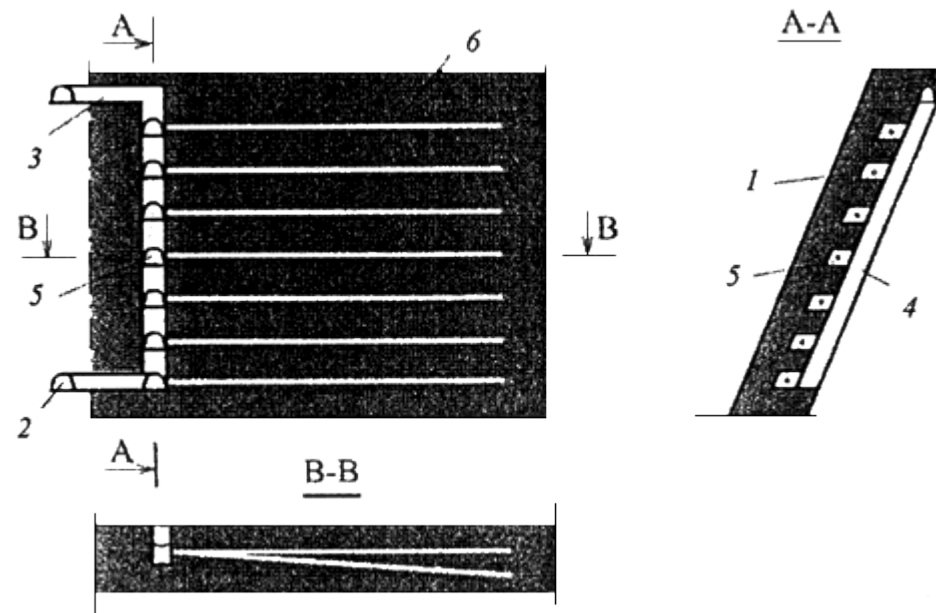
Рис.3. Схема дегазации разрабатываемого пласта скважинами, пробуренными по простиранию пласта из подэтажных камер: 1 - разрабатываемый пласт; 2 - полевой штрек; 3 - промежуточный квершлаг; 4 - скат; 5 - камера; 6 - дегазационная скважина
