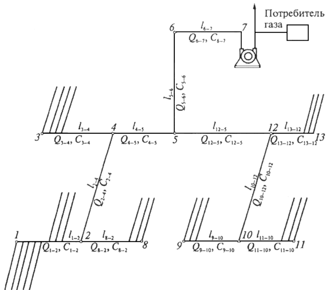
Рис.1. Схема для расчета газопроводов
