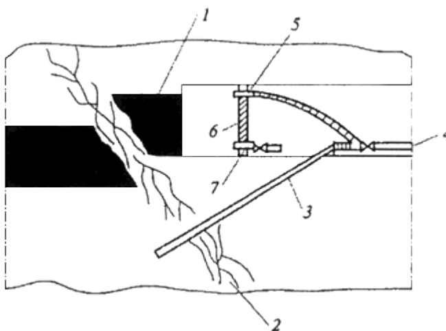
Рис.2. Схема извлечения метана из суфлярных трещин средствами дегазации путем бурения скважин и возведения изолирующей забой перемычки: 1 - угольный пласт; 2 - геологическое нарушение; 3 - скважина; 4 - газопровод; 5 - шланг для отвода газов; 6 - перемычка; 7 - труба с вентилем для слива воды
