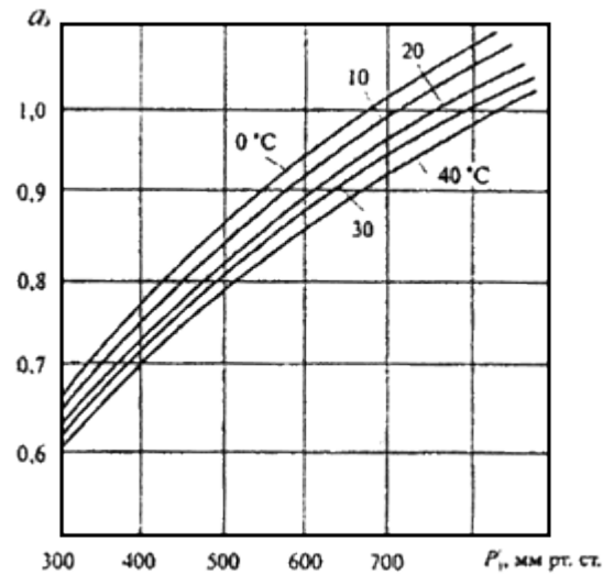
Рис.4. Определение поправочного коэффициента \alpha_3
