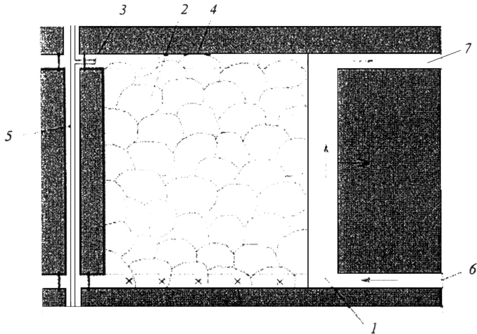
Рис.4. Схема дегазации выработанного пространства с использованием дегазационного газопровода во фланговой выработке:
