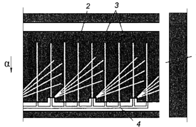
Рис.11. Схема дегазации пласта параллельными и веерными, ориентированными на очистной забой, скважинами:
