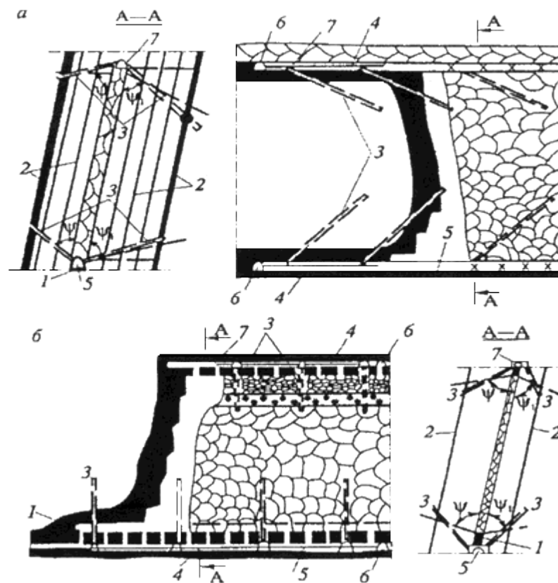
Рис.6. Схема дегазации крутых сближенных пластов скважинами, пробуренными из выработок разрабатываемого пласта:
