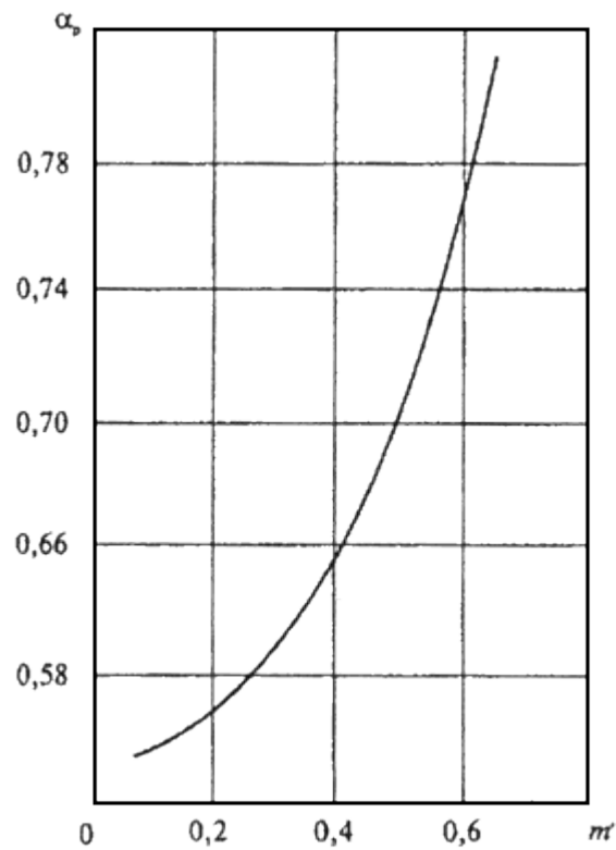
Рис.5. Зависимость коэффициента расхода \alpha_p от m' = \frac{d_0^2}{d^2}
