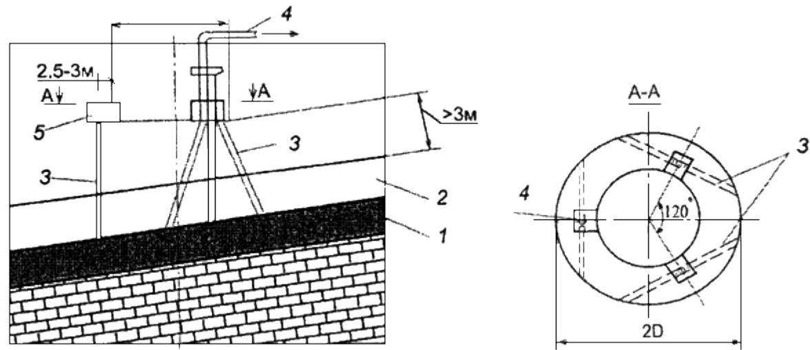
Рис.1. Схема дегазации газоносного массива при проходке вертикальных выработок:
