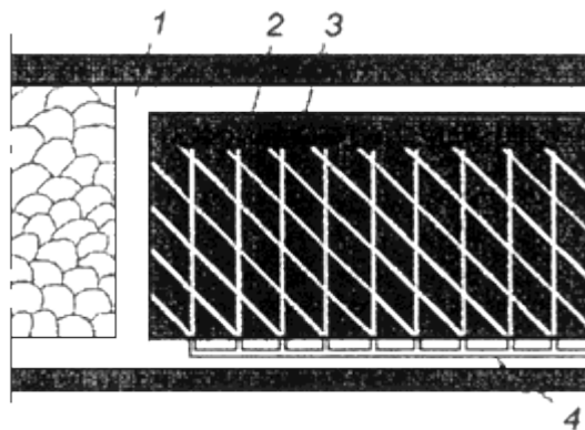
Рис.10. Схема дегазации угольных пластов перекрещивающимися скважинами, пробуренными из конвейерной выработки:
