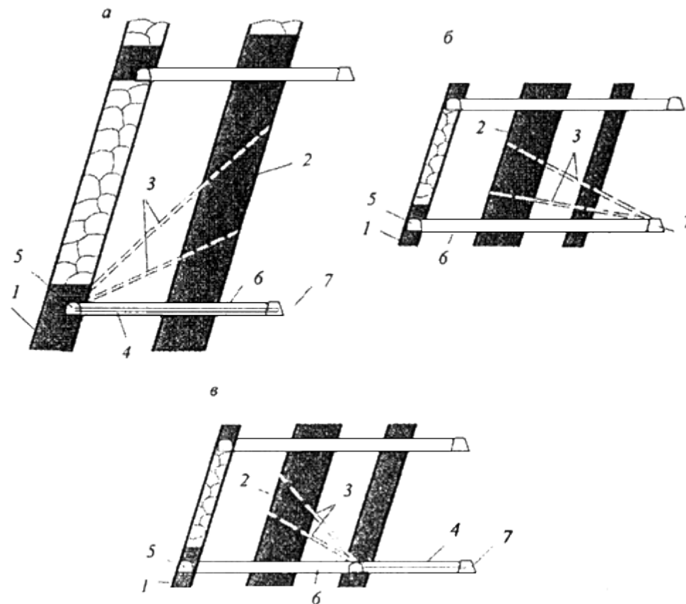
Рис.1. Схема дегазации надрабатываемого крутого пласта скважинами, пробуренными веером вкрест его залегания:
