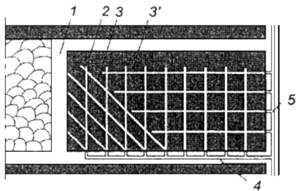
Рис.9. Схема дегазации угольных пластов при ограниченных возможностях буровой техники:
