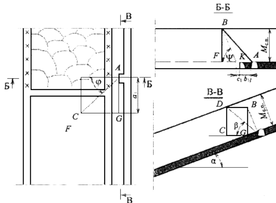
Рис.7. Графическое определение параметров дегазационных скважин, буримых на подрабатываемый пласт из поддерживаемой выработки в лавах по падению
