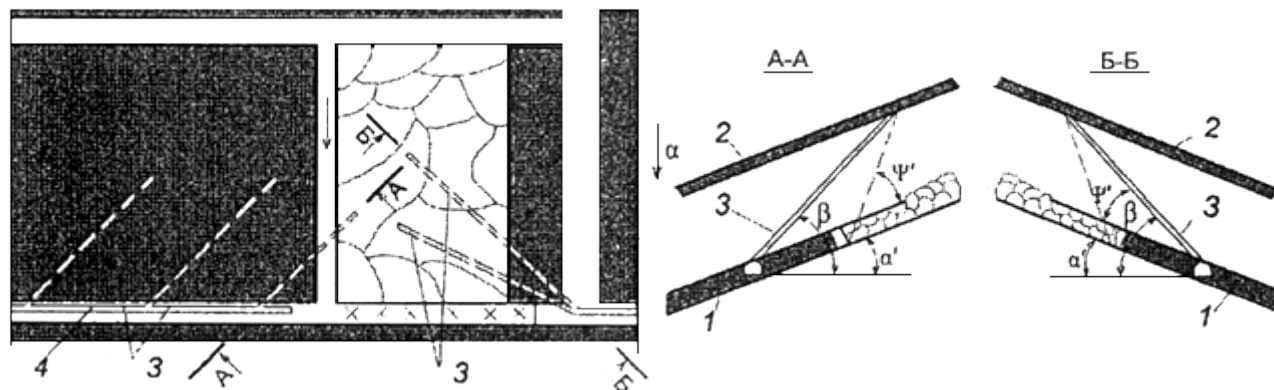
Рис.5. Схема дегазации подрабатываемого пласта скважинами в период первичной посадки основной кровли:
