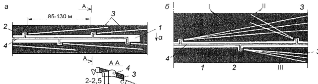
Рис.5. Схема дегазации пласта барьерными скважинами:
