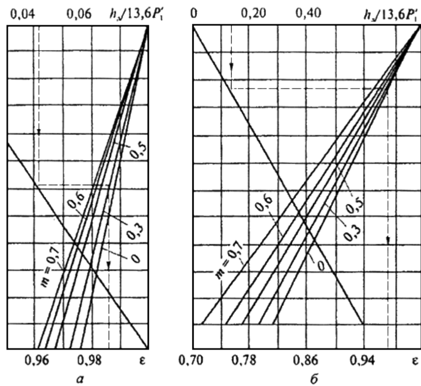
Рис.3. Определение коэффициента \varepsilon при малых (а) и при больших (б) значениях h_d / 13.6 P_1'
