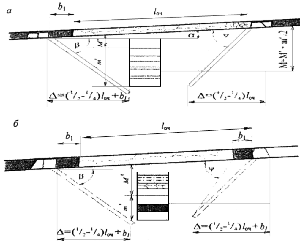
Рис.1. Схемы дегазации надрабатываемой толщи горных пород:
