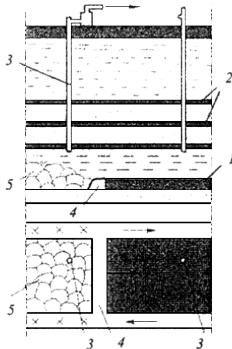
Рис.2. Схема дегазации подрабатываемых пластов скважинами, пробуренными с поверхности: 1 - разрабатываемый пласт; 2 - сближенные пласты; 3 - скважина; 4 - очистной забой; 5 - выработанное пространство
