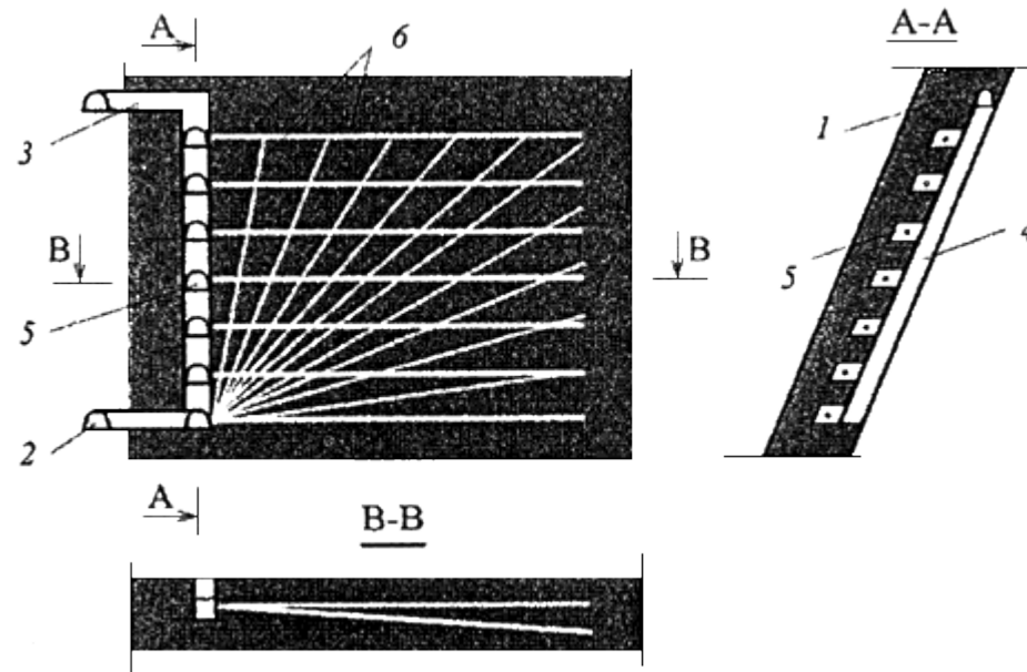
Рис.4. Схема дегазации разрабатываемого пласта перекрещивающимися скважинами, пробуренными из подэтажных камер и из нижнего подэтажного штрека:
