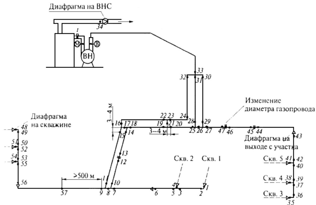
Рис.1. Схема расположения пунктов замера параметров газозвушных потоков при проведении вакуумно-газовой съемки
