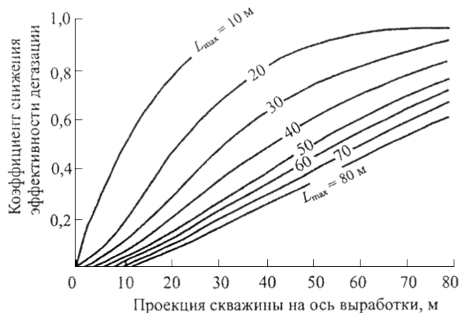
Рис.9. Снижение эффективности дегазации сближенных пластов на участках, обрабатываемых с погашением выработок за лавой
