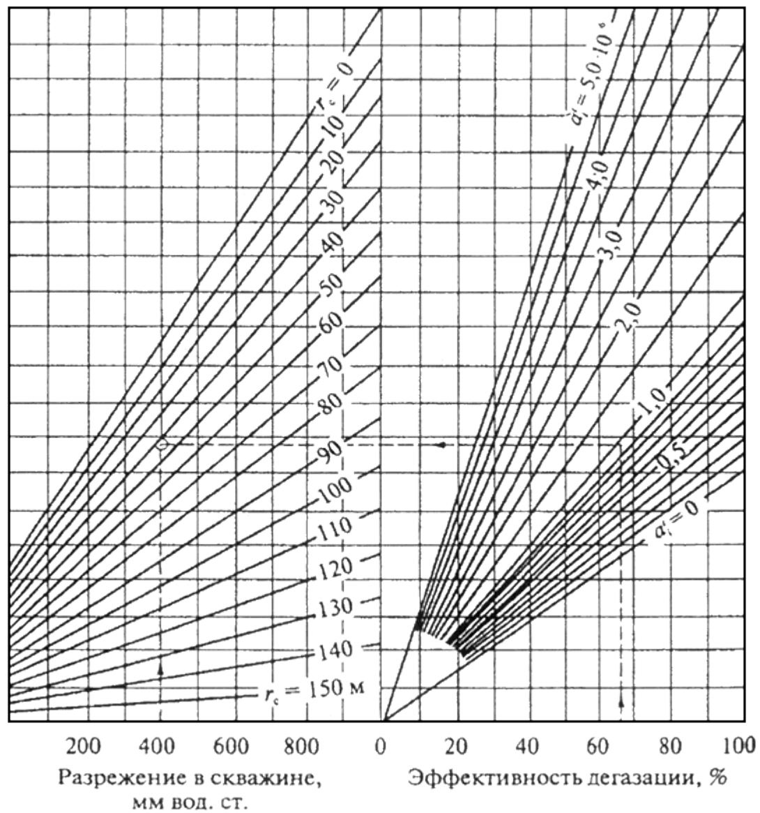
Рис.8. Определение расстояния между скважинами при их бурении на подрабатываемые угольные пласты 16. При бурении скважин из выработок, погашаемых за лавой, вводится коэффициент снижения эффективности дегазации, определяемой по
