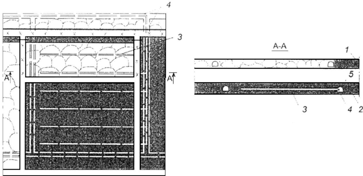
Рис.3. Схема дегазации надрабатываемого угольного пласта пластовыми скважинами:
