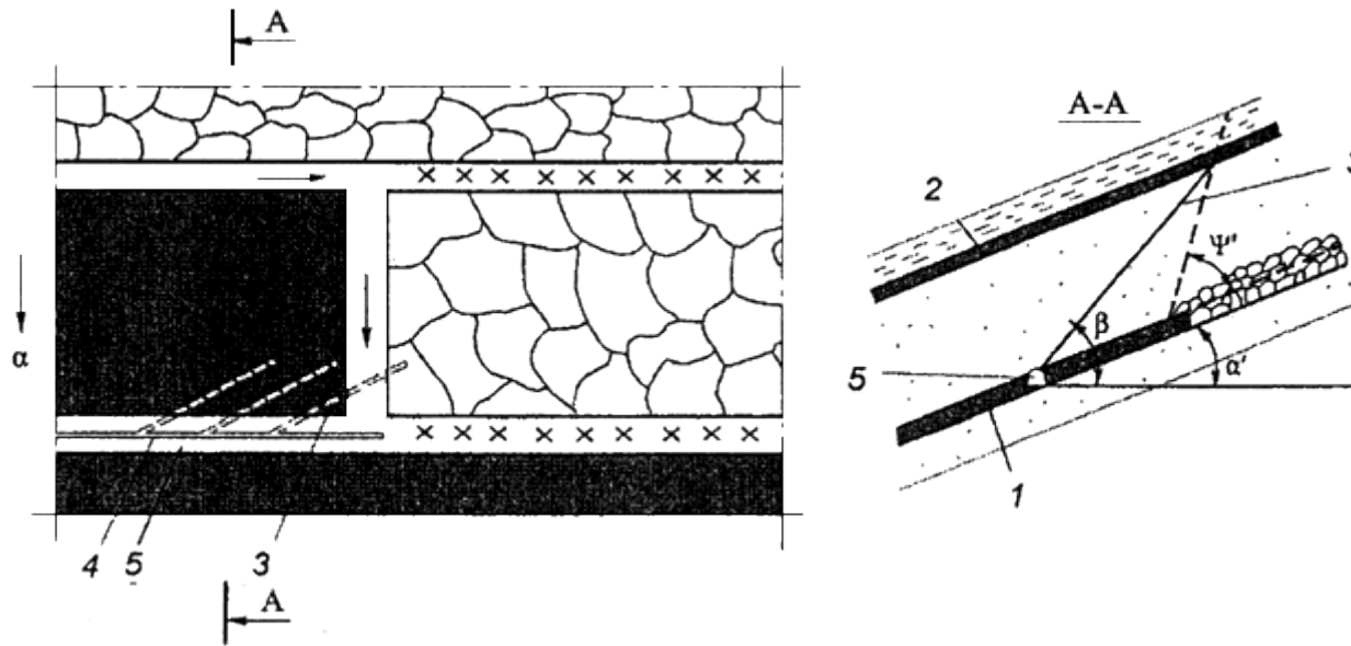
Рис.3. Схема дегазации подрабатываемого пласта скважинами, пробуренными навстречу движущемуся очистному забою из погашаемой за лавой выработки (схема 3):
