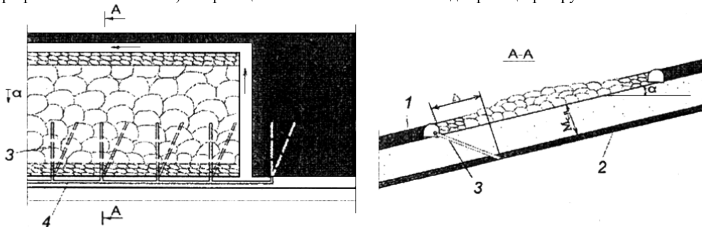
Рис.2. Схема дегазации надрабатываемого пласта скважинами, пробуренными из поддерживаемой за лавой откаточной выработки:
