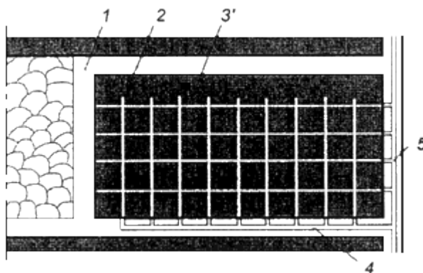
Рис.8. Схема дегазации угольного пласта при бурении параллельных и сверхдлинных направленных на очистной забой скважин:
