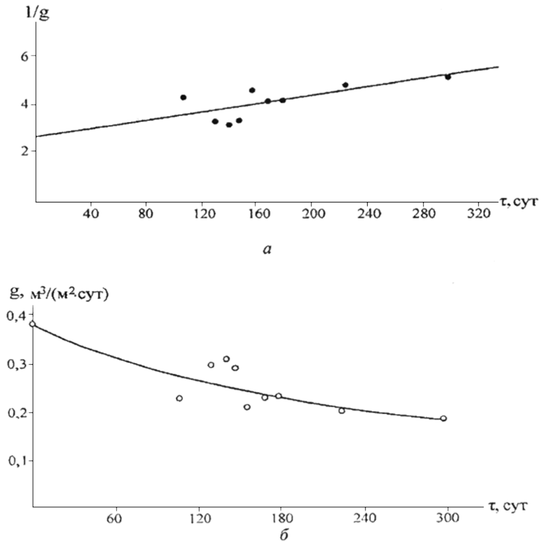
Рис.2. Графики зависимости удельного метановыделения из угольных пластов в скважины
