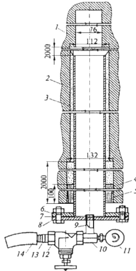
Рис.2. Приспособление для контроля герметичности скважины:
