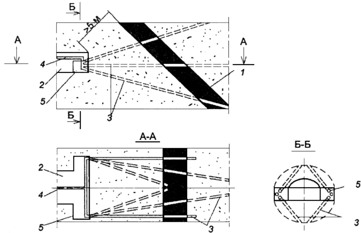
Рис.2. Схема дегазации газоносного массива при вскрытии квершлагом:
