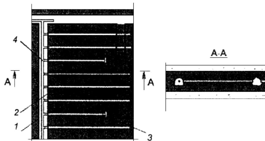
Рис.18. Схема дегазации с предварительным гидроразрывом пласта через скважины, пробуренные из пластовой выработки:
