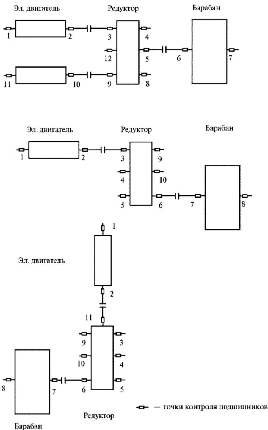
Рис.1. Схема контроля вибрации
