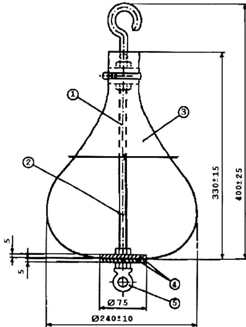
Рис.3. Маятник для нежесткого удара:
