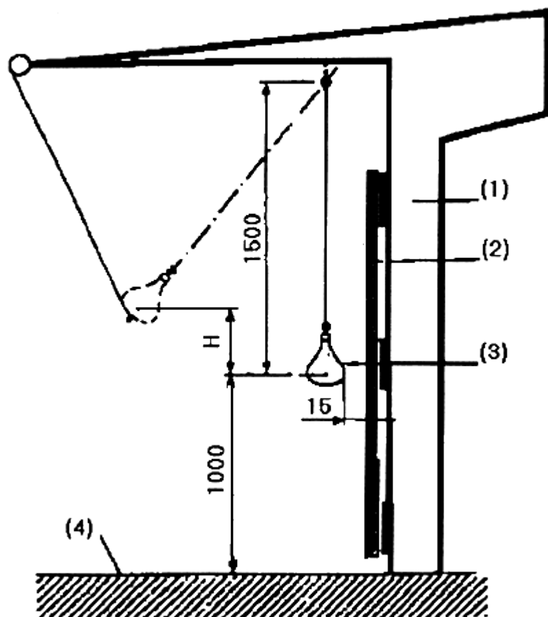
Рис.1. Испытательный стенд:
